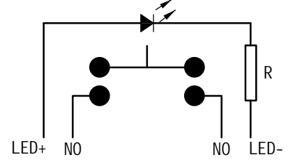
电气原理图
