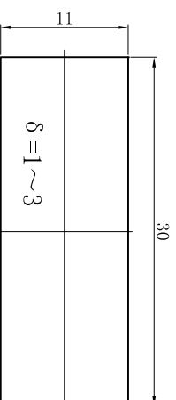
安装面板尺寸 PANEL CUT-OUT
